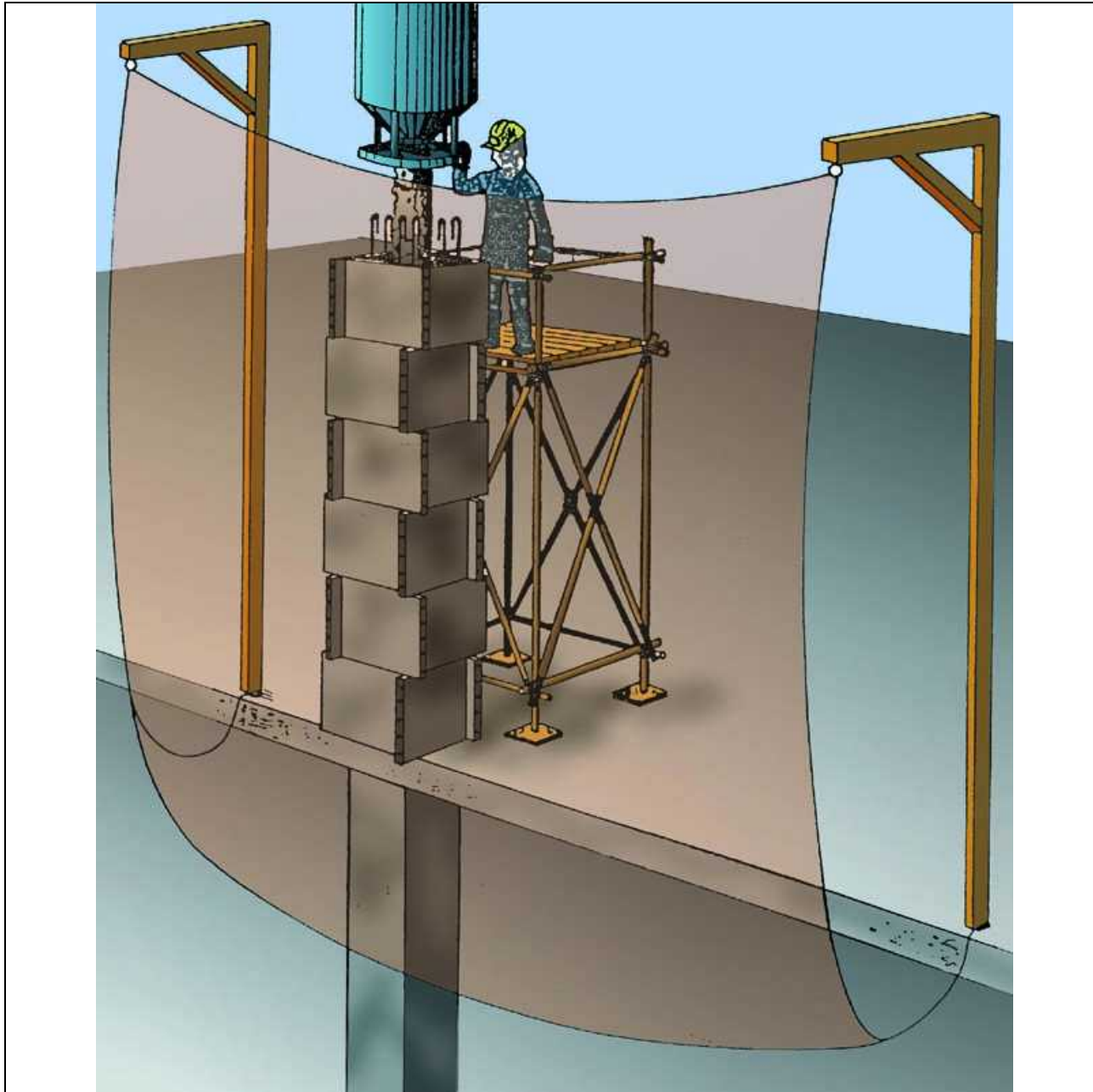
PERSPECTIVA
