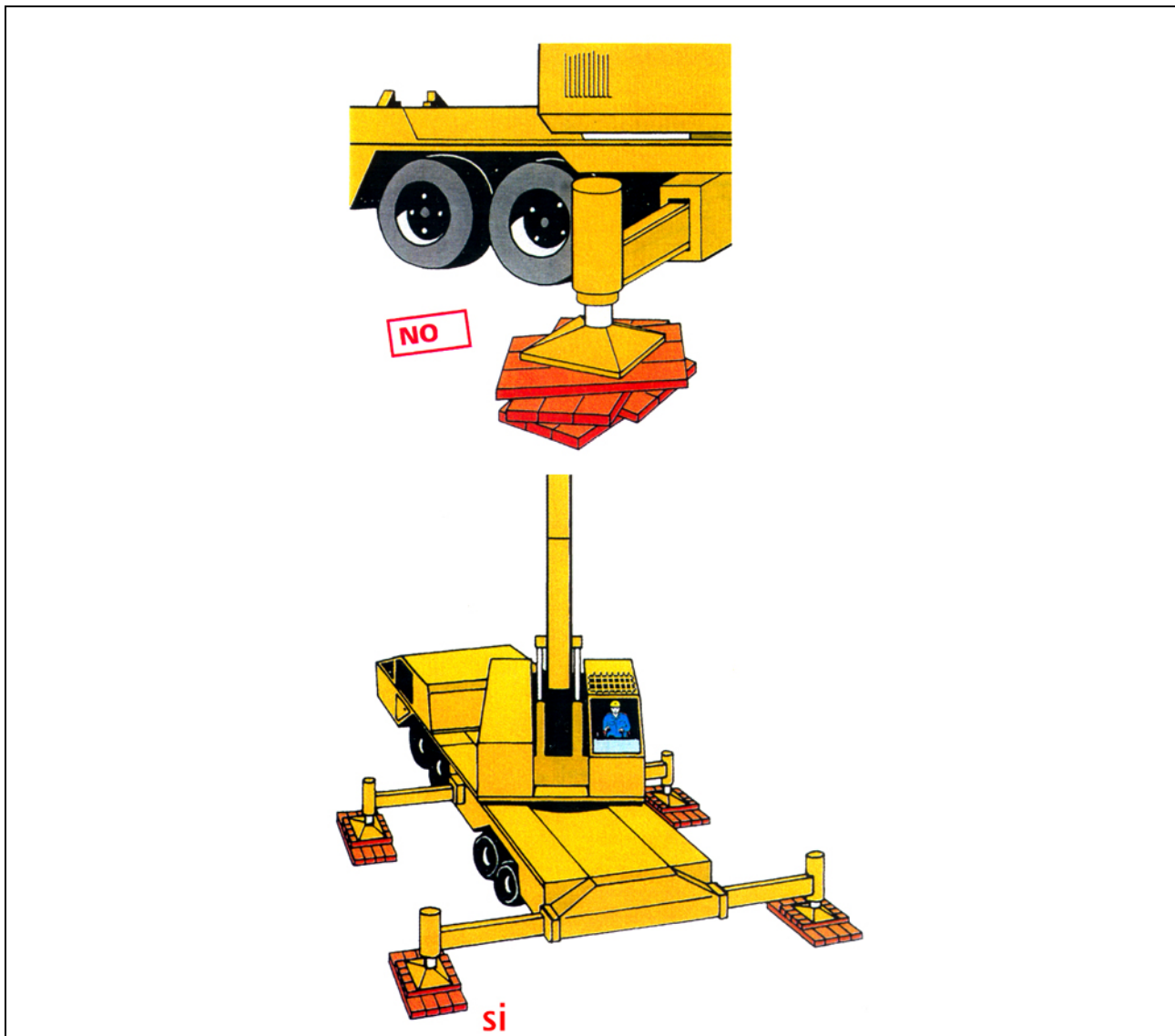
Col·locació estabilitzadors recolçaments
